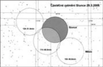
Průběh částečného zatmění Slunce 29. 3. 2006
