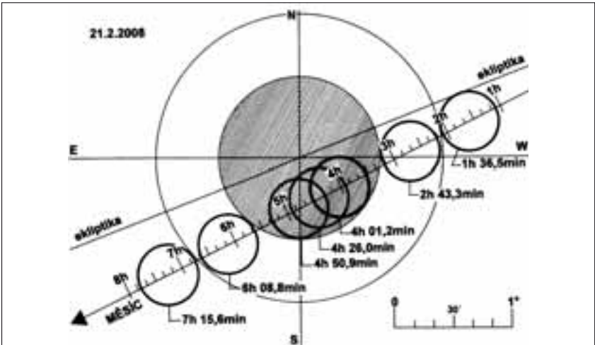
Zatmění Měsíce 21. února 2008. (Převzato z Hvězdářské ročenky 2008.)
